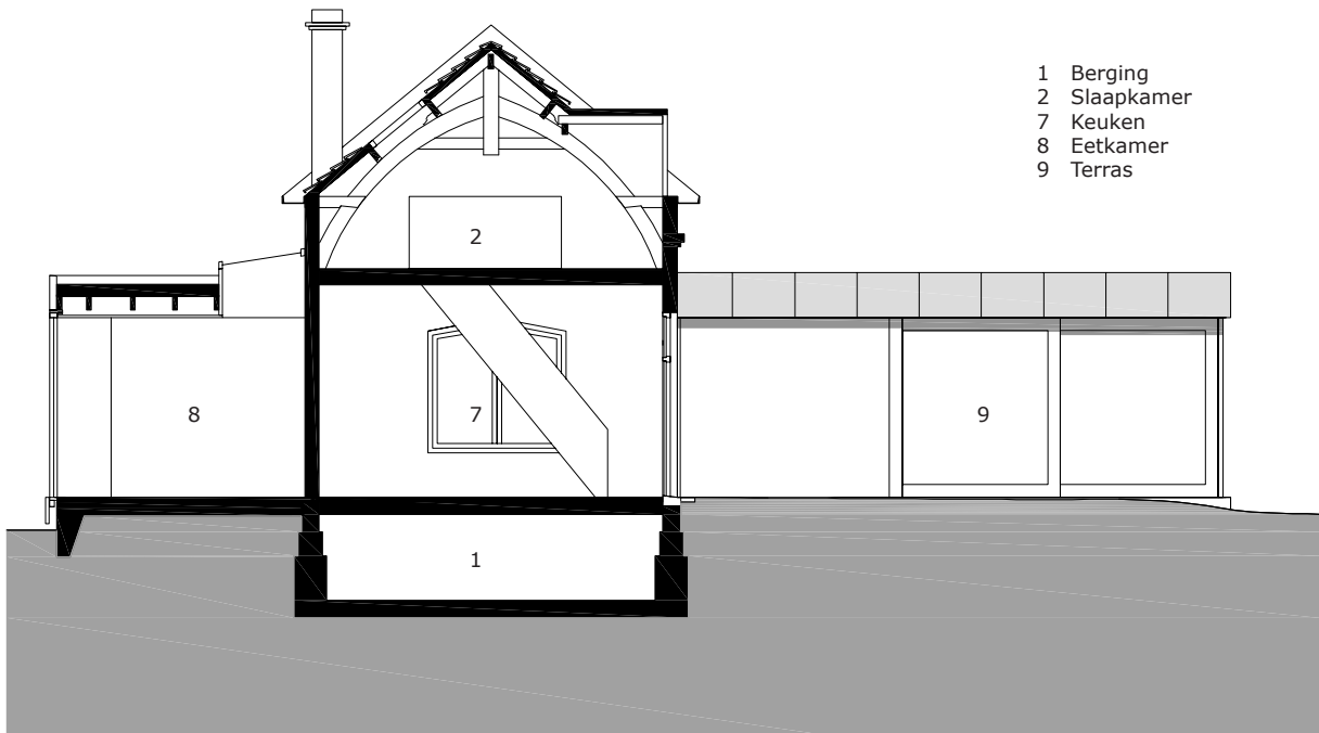
doorsnede BB
