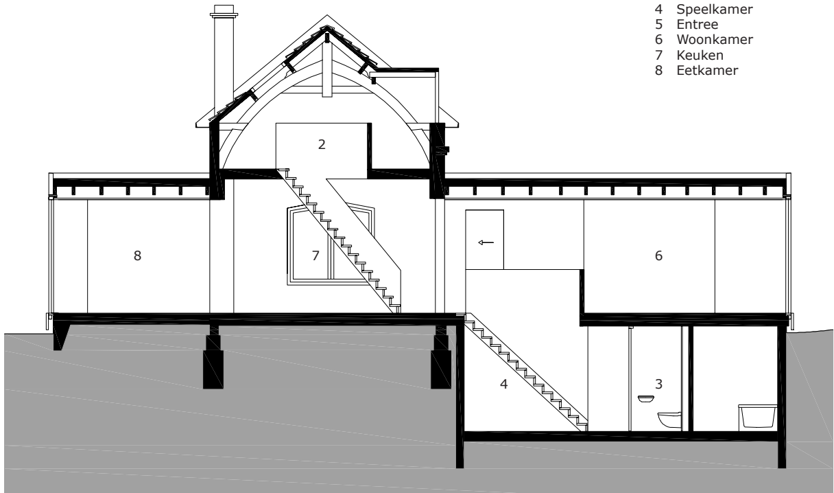
doorsnede AA
